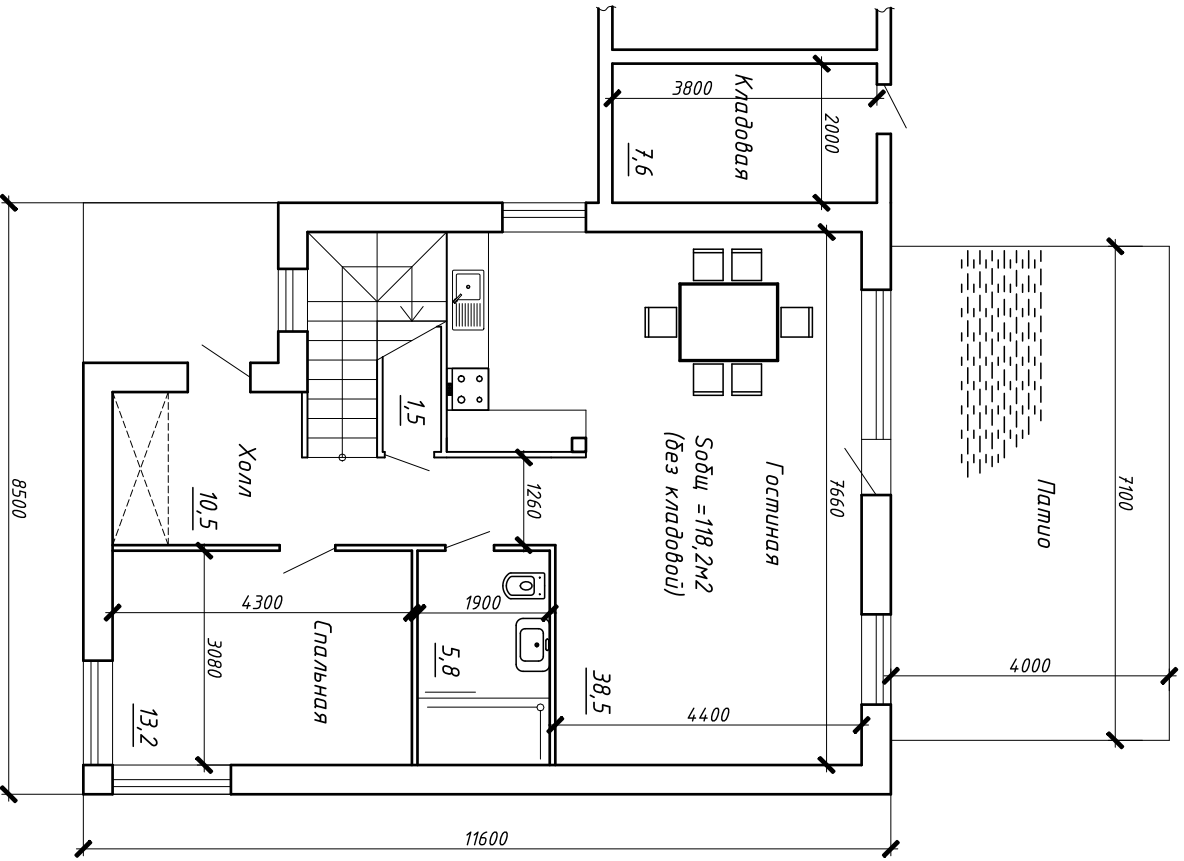
План 1 этажа
