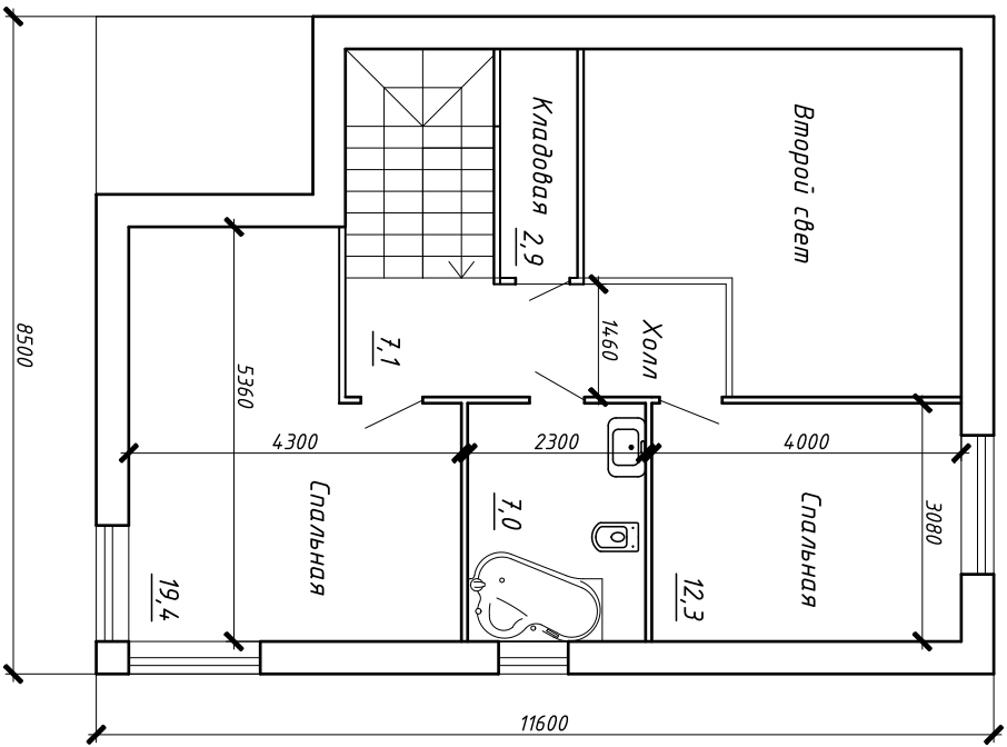
План 2 этажа
