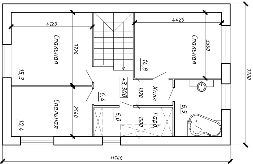
План 2 этажа
